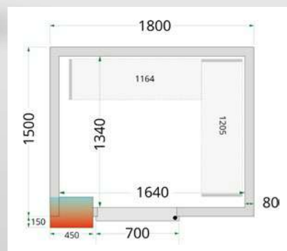
Rozměry CR 180×150×220 (80 mm)
